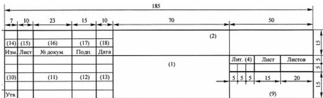
Рис. 1. Форма основной надписи для первого листа текстового документа.
