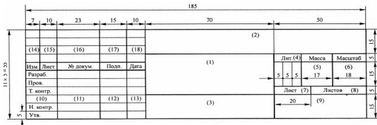
Рис. 3. Форма основной надписи для чертежей.
