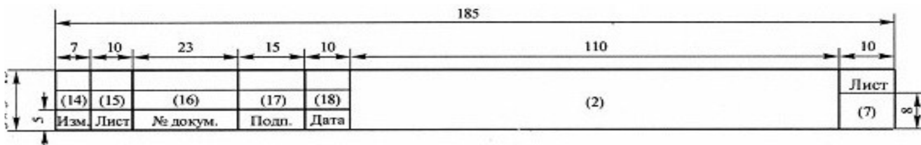
Рис. 2. Форма основной надписи для последующих листов.
