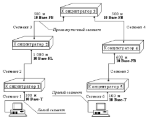
Рисунок 2.1 - Пример сети Ethernet, состоящей из сегментов различных физических стандартов распространения сигнала вдоль кабеля сегмента, которая зависит от длины сегмента и вычисляется путем умножения времени распространения сигнала по одному метру кабеля (в битовых интервалах) на длину кабеля в метрах.
